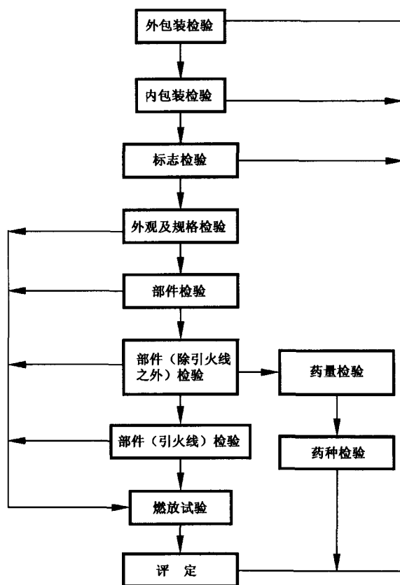
图1 罗马烛光检验评定流程
